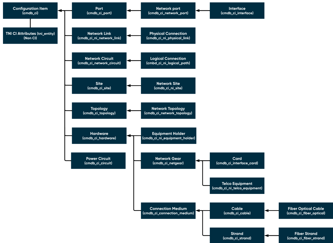
네트워크 인벤토리 데이터 모델
