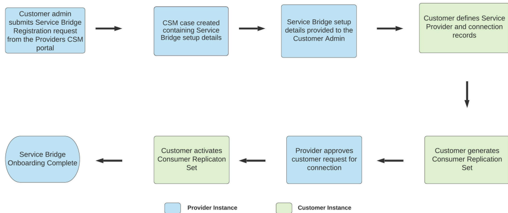
고객 통합 온보딩
